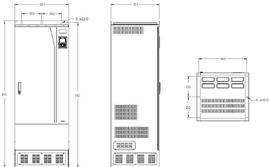
Рисунок С.13 Схема для напольного монтажа приводов 355G/400P-500G
