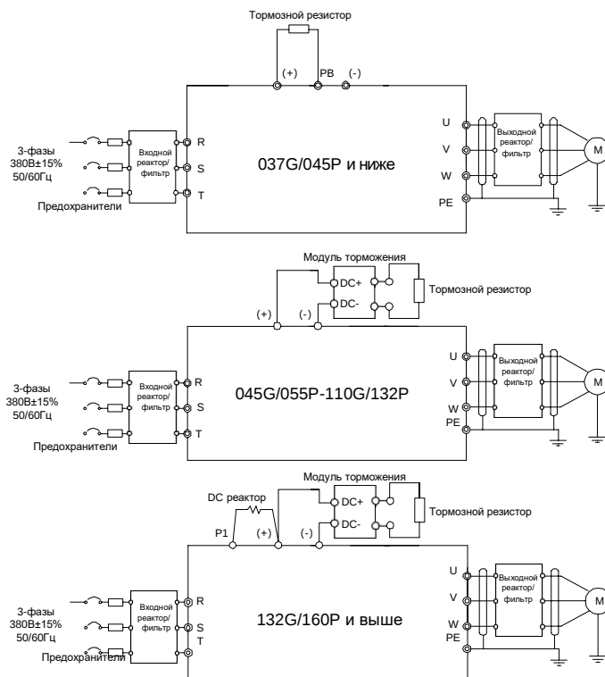
Рис 4.7 Схема подключения силовой цепи
