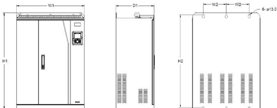
Рисунок С.8 Схема настенного монтажа приводов 220G/250P-315G/350P
